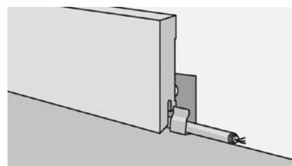
Рис. 113. После укладки пола нужно вынуть фиксирующие клинья, а расширительные зазоры закрыть декоративным плинтусом. Плинтус крепится только к стене. Не допускается крепление плинтуса к напольному покрытию. Рекомендуем использовать для крепления специальные клипсы для плинтуса.
