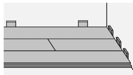
Рис. 106. Перед приклеиванием проведите подрезку и пробную сборку трех первых рядов без клея. с каждой стороны ряда необходимо оставить компенсационный зазор (8-10 мм.), в который устанавливаются расширяющие клинья.
