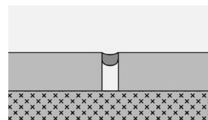
Рис. 33. Площадь контакта сварочного шнура и покрытия слишком маленькая. При этом прочность сваренного шнура примерно 10-15 N/см.
