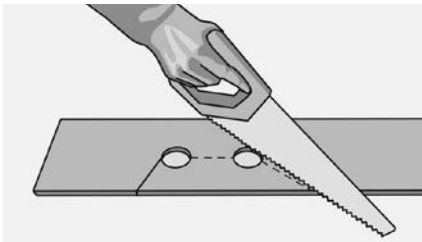
Рис. 102. Если длинная сторона доски упирается в трубу, просверлите отверстие диаметром, превышающим диаметр трубы примерно на 16 мм, для создания компенсационного зазора вокруг трубы. Отметьте карандашом линию отреза. Отпилите кусок доски, который будет располагаться за трубой ближе к стене.
