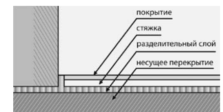
Рис. 14. Стяжка на разделительном слое
