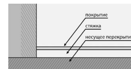
Рис. 13. Соединительная стяжка
