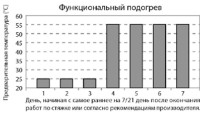
Рис. 15. Функциональный подогрев
