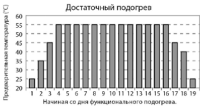
Рис. 16. Достаточный подогрев
