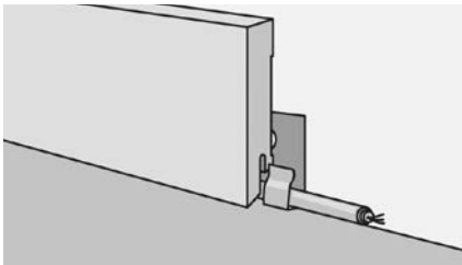
Рис. 104. После укладки пола нужно вынуть фиксирующие клинья, а расширительные зазоры закрыть декоративным плинтусом. Плинтус крепится только к стене. Не допускается крепление плинтуса к напольному покрытию.
