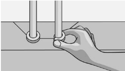
Рис. 103. Подгоните доску, чтобы она встала на место, вклейте на место отпиленный кусок, установите распорку между стеной и доской и закройте зазор вокруг трубы специальным кольцом.
