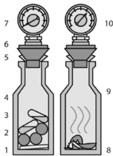
Рис. 10. Прибор CM (измерение при помощи карбидно-кальциевого метода)
